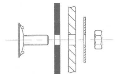
Elevatorbekerbevestiging met vlakke boutgaten
