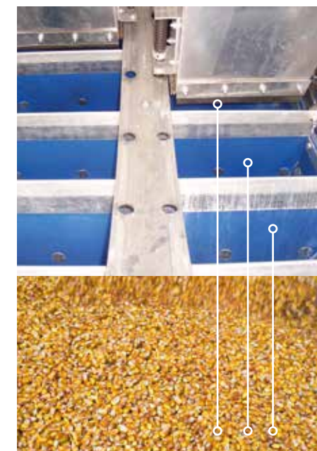
Bekleding productverdeeklep in graan verwerkende industrie – Blue-Ox®
