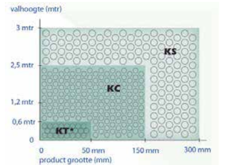
REDI-LINER™ selectie schema
