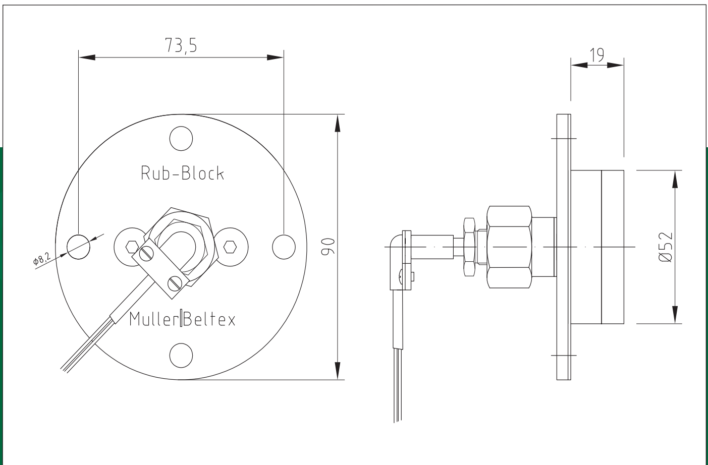
Zijaanzicht
