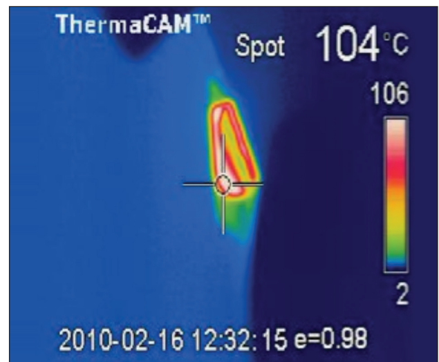
Warmtebeeldfoto RB100DN .
