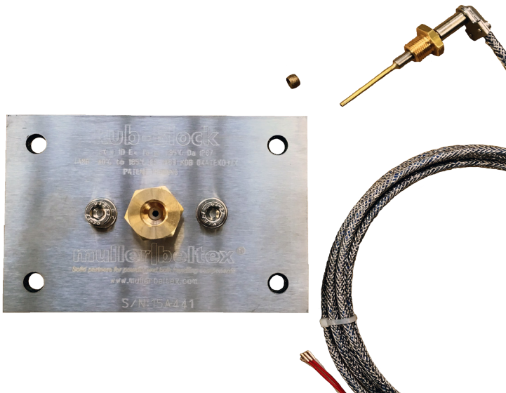
Step 1: Begin met bovengenoemde drie componenten.
